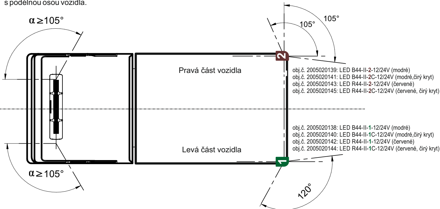
Obr. 1: Varianta A - montáž při použití světelné soupravy a dvou zadních rohových svítidel LED x 44-II.
