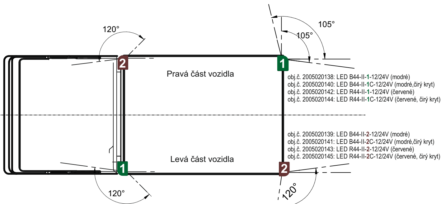
Obr. 2: Varianta B - montáž při použití dvou předních a dvou zadních rohových svítidel LED x 44-II.
