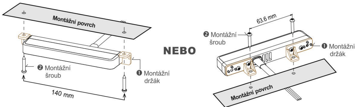
Obr. 3: Montáž svítidla s uchycením na držáky v "L" tvaru
