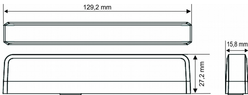
Obr. 1: Rozměry svítidla
