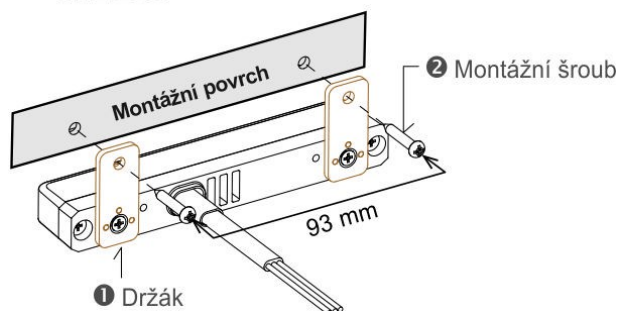
Obr. 2: Montáž svítidla na držáky ve tvaru obdélníku
