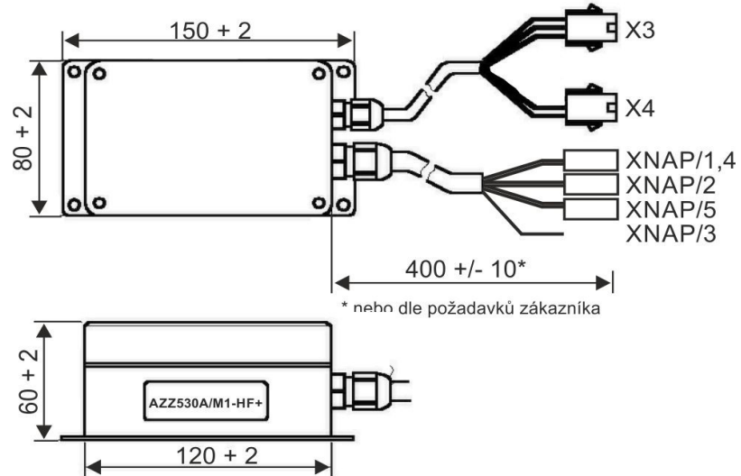
Obr. 1: Zesilovač
