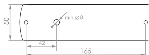
Obr. 2: Rozměrový náčrtek svítidla
