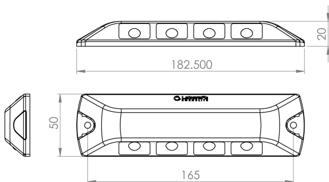
Obr. 1: Rozměry svítidla
